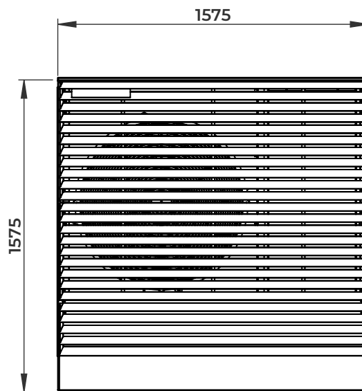
VORDERSEITE
