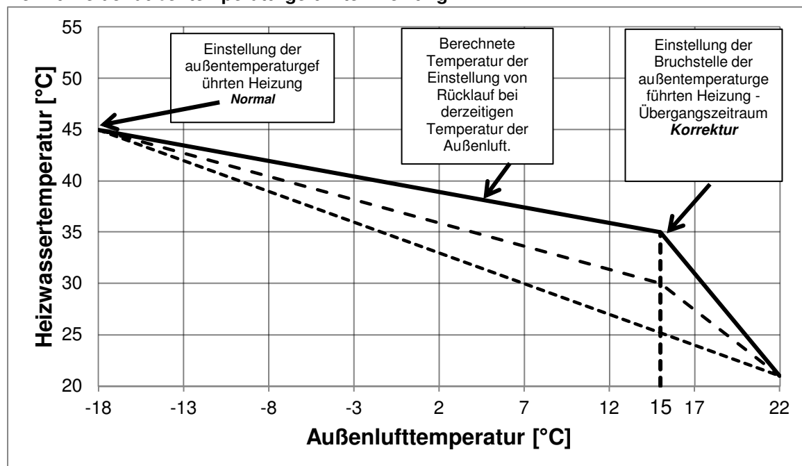
Heizkurve der außentemperaturgeführten Heizung
