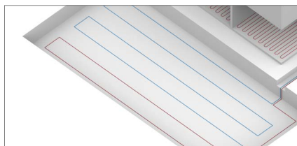
ZEMLJA/VODA - HORIZONTALNI ZEMELJSKI KOLEKTOR
